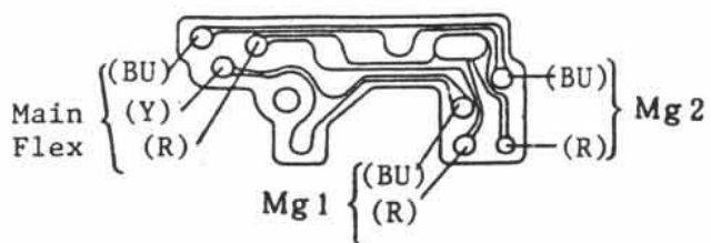
22 Wiring
